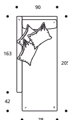
Art. 9059 SCHLUSSECKELEMENT 205 li./re. MIT 3 RÜCKENKISSEN 50x50 90 X 205 X h. 80 cm
