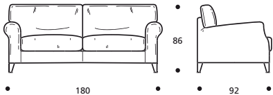
Art. 8620 3-SITZER-BETTISOFA, KLEIN 180 180 x 92/224 x h. 86/96 cm FEDERKERNMATRATZE: 115 x 192 x h.13 cm Stoffbedarf h.140 cm: 12,30 m
