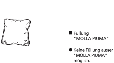
Art. 0118 KORDELKISSEN 45x45 45/48 x 45/48 x h.1/15 cm Stoffbedarf h.140 cm: 0,70 m
