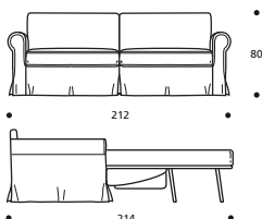
Art. 9043 3-SITZER-BETTISOFA 212 212 X 92/214 X h. 80 cm
