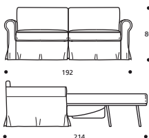
Art. 9042 3-SITZER-BETTISOFA 192, KLEIN 192 X 92/214 X h. 80 cm
