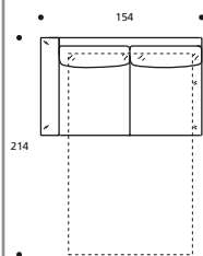
Art. 9045 BETTELEMENT 154 li./re. 154 X 92/214 X h. 80 cm
