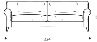
Art. 8620 3-SITZER-BETTISOFA, KLEIN 180 180 x 92/224 x h. 86/96 cm FEDERKERNMATRATZE: 115 x 192 x h.13 cm Stoffbedarf h.140 cm: 12,30 m
