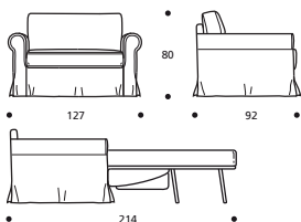
Art. 9040 SESSEL 127 MIT BETTEINBAU 127 X 92/214 X h. 80 cm
